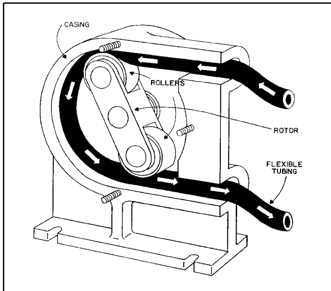
Fig. 11. Peristaltic pump.
