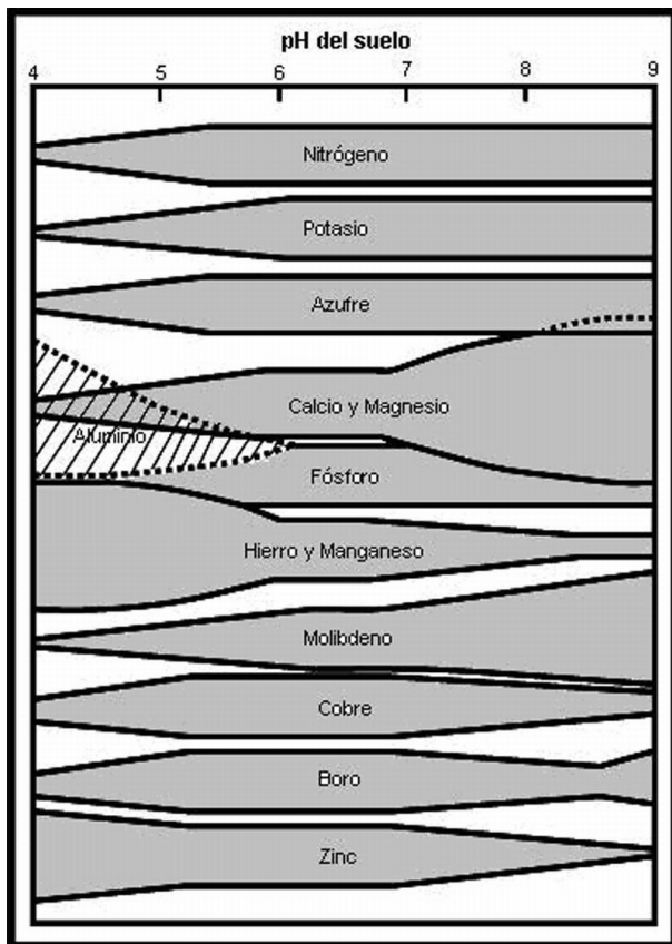
Figura 3. Relación entre pH del suelo y disponibilidad de nutrientes para la planta. Para cada elemento, entre más ancha la banda, más disponibilidad de elemento. Adaptado de Brady y Weil, 1999.
