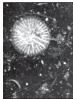
Micrasterias
