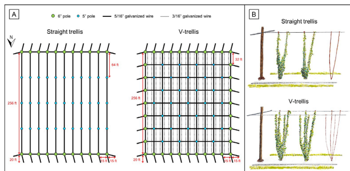
Figura 3. Diseños de tutorado recto y en "V" usados para el campo de lúpulo de GCREC: A) planos del tutorado y B) diagramas del tutorado. Créditos: Shinsuke Agehara y Aleyda Acosta-Rangel, UF/IFAS
